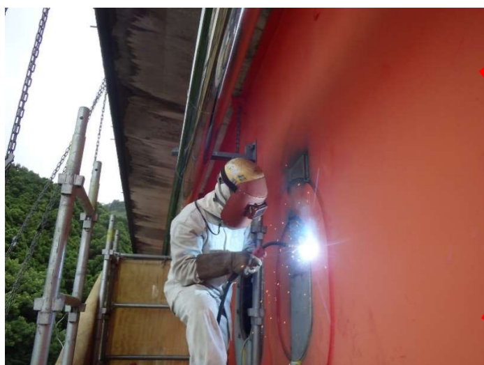
ボルト及び溶接で補強部材を接合
