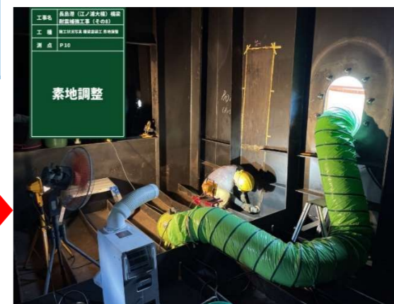
ジャッキアップ補強部材取付部素地調整
